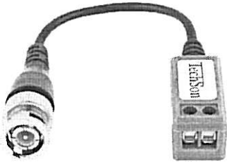
TechSon SP111/2R. Egy csatornás, rögzítő oldali passzív videó balun.
